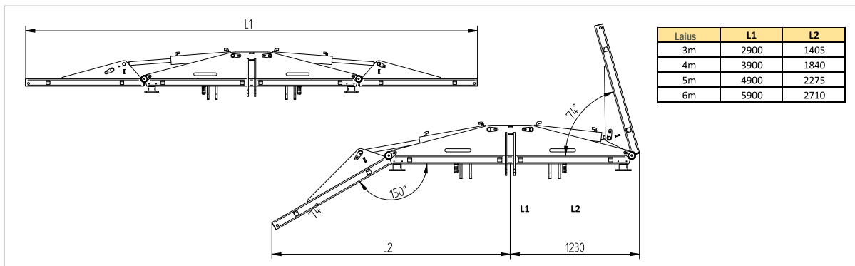
Kahe külghõlma kaudu pidevalt reguleeritav puhastuslaius, lisavõre (valikuline)
