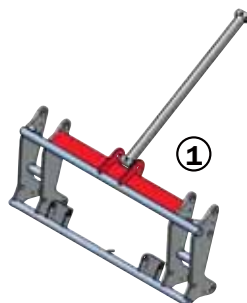
Kiirvahetusraam, hüdrauliliselt lukustatav
