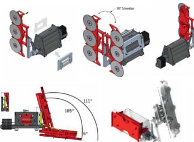
Vasakpoolne kinnitus teleskooplaaduril
