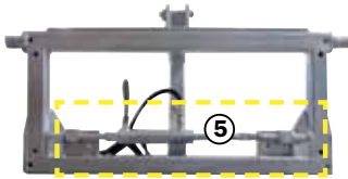
③+④ Kolmpunkt-kinnituse adapter, hüdrauliline lukustatav
