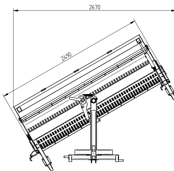
Kolmepunktkonks esi- ja tagahaakeseadmele
