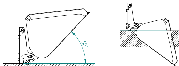
Suur kallutusnurk ideaalseks täitmiseks ja tühjendamiseks
