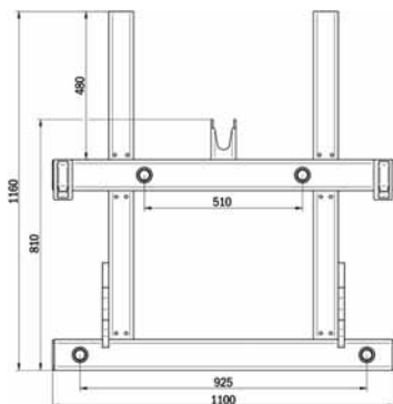
Kõrgenduse ja 4 ümarpalliipiigiga versioon (2 piiki standardvarustuses)
